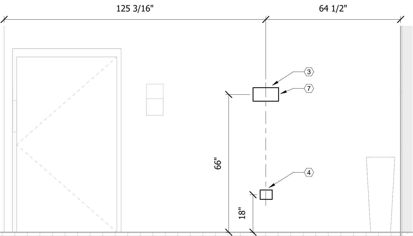
FIRE ROOM 104B SCALE: 1/2" = 1'-0"
