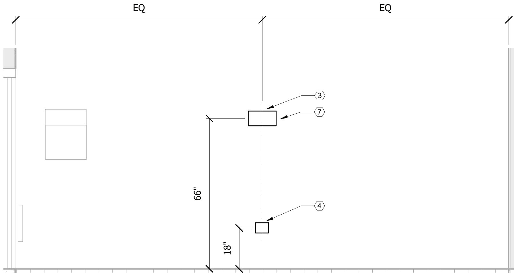
FIRE ROOM 104C SCALE: 1/2" = 1'-0"
