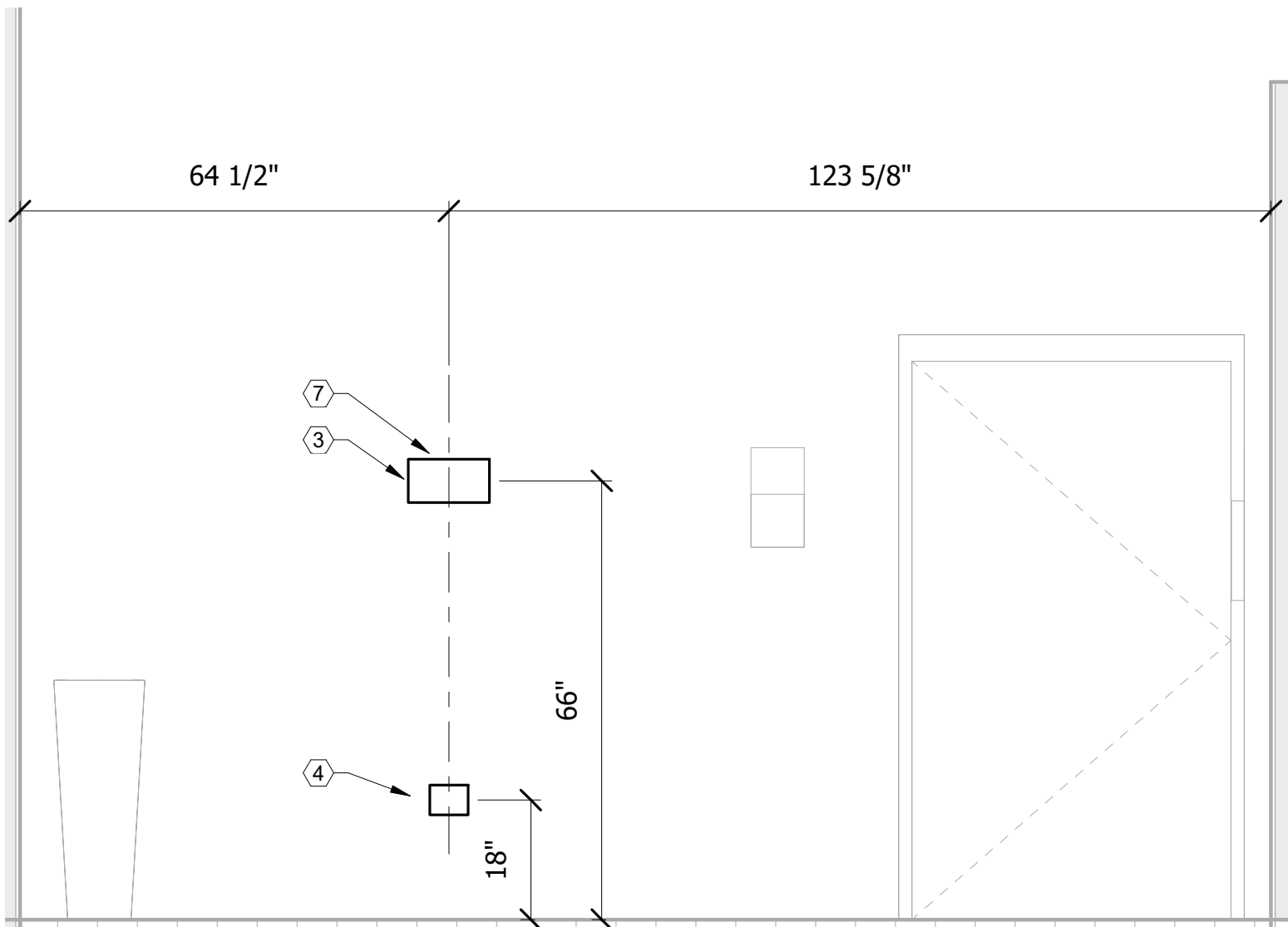
FIRE ROOM 104A SCALE: 1/2" = 1'-0"
