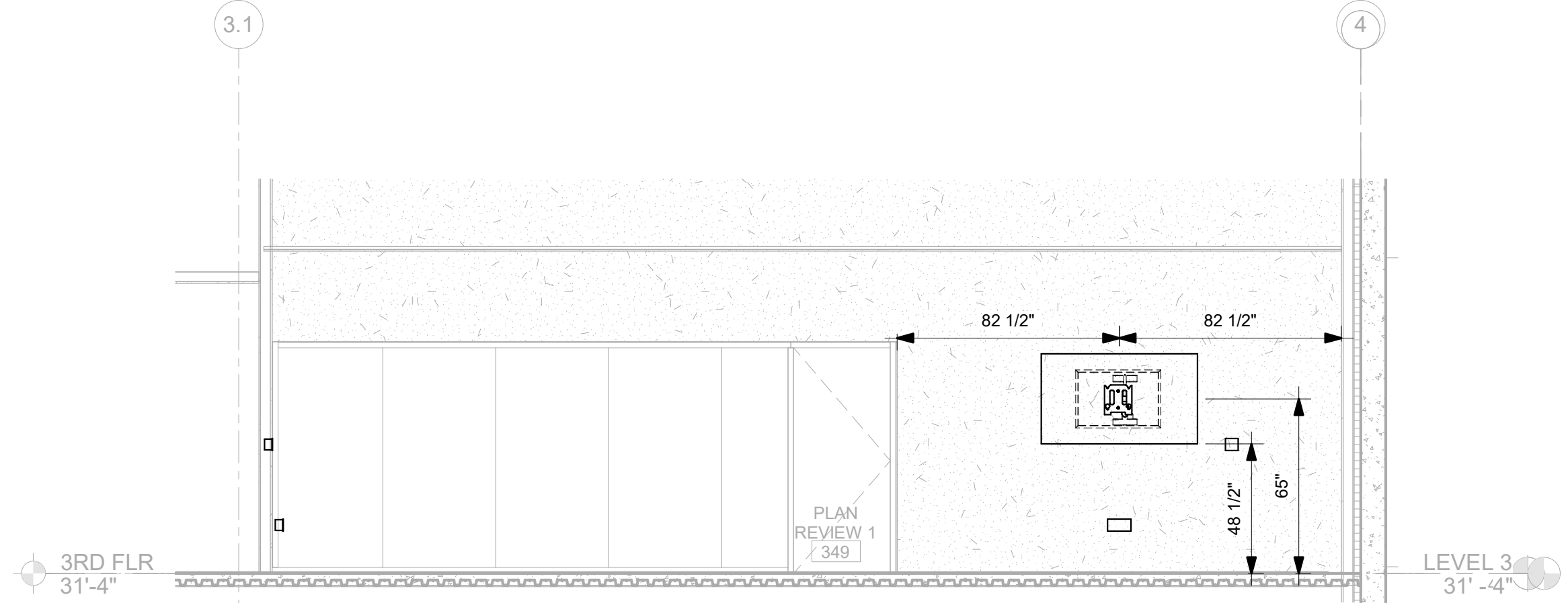
1 AV-306 AV ELEVATION DETAILS - PLAN REVIEW 1 EAST WALL 1/4" = 1'-0" 2 AV-306 AV ELEVATION DETAILS - PLAN REVIEW 1 SOUTH WALL 1/4" = 1'-0"
