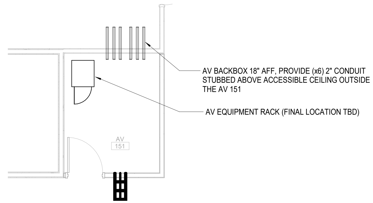
4 AV ROOM 151 - ENLARGED PLAN AV-201 1/4" = 1'-0"
