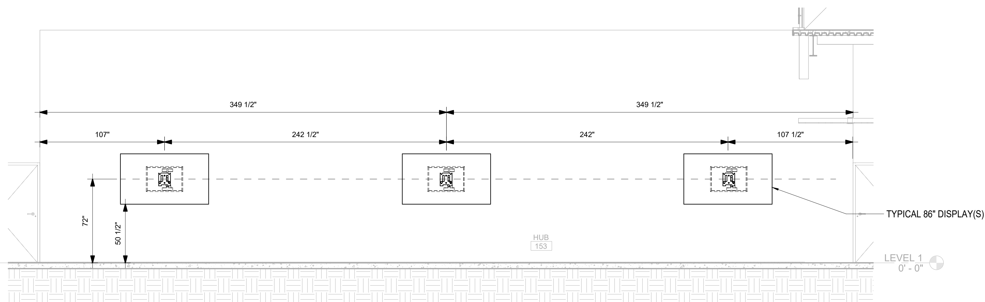
7 AV-301 AV ELEVATION DETAILS - PROJECTION SCREEN - PROJECTOR 1/4" = 1'-0" 8 AV-301 AV ELEVATION DETAILS - CONF 138 1/4" = 1'-0"
