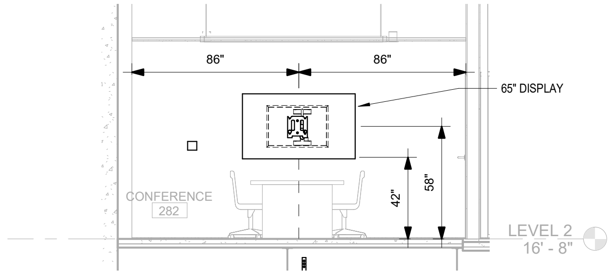
3 AV ELEVATION DETAILS - CONFERENCE ROOM 282 1/4" = 1'-0" AV-305
