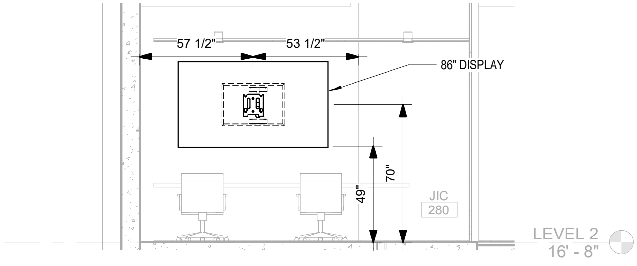
1 AV-305 AV ELEVATION DETAILS - JIC 280 1/4" = 1'-0"
