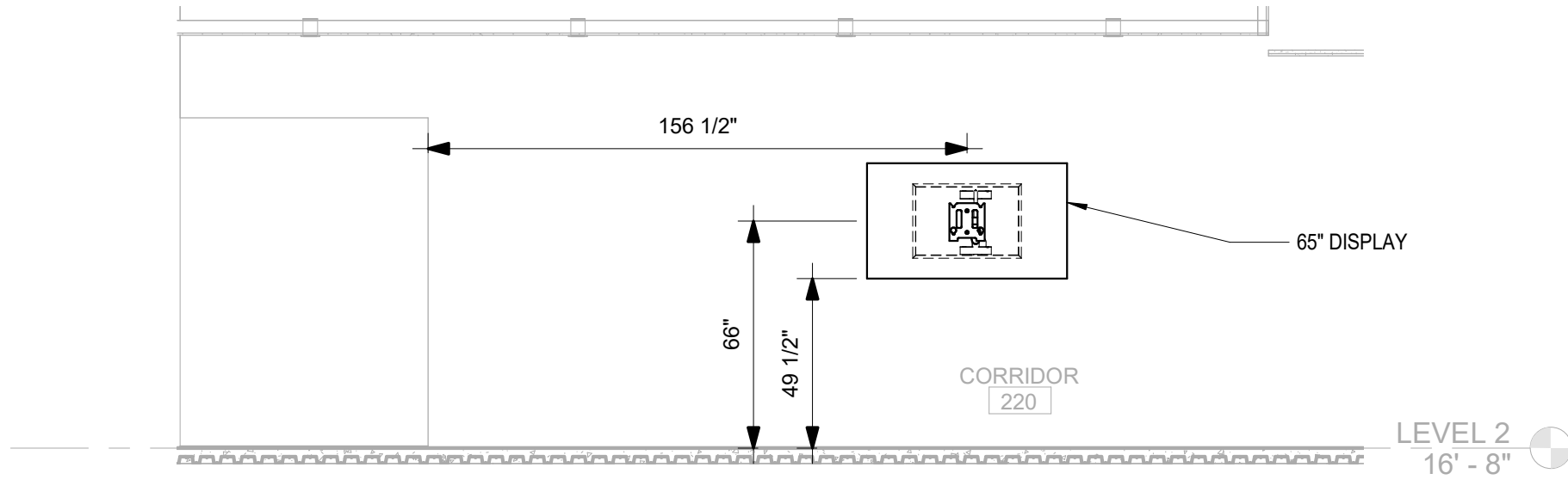
1 AV ELEVATION DETAILS - CORRIDOR 220 AV-303
