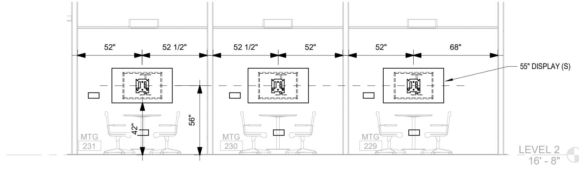
5 AV ELEVATION DETAILS - MTG ROOM (S) 1/4" = 1'-0" AV-303
