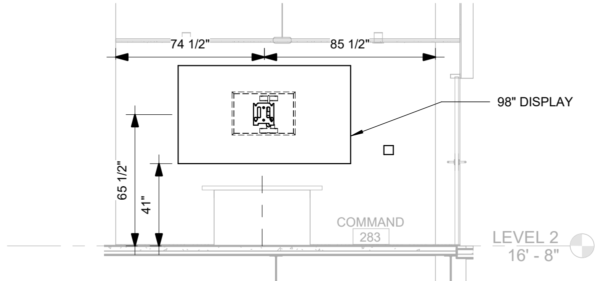
4 AV ELEVATION DETAILS - COMMAND 283 1/4" = 1'-0" AV-305
