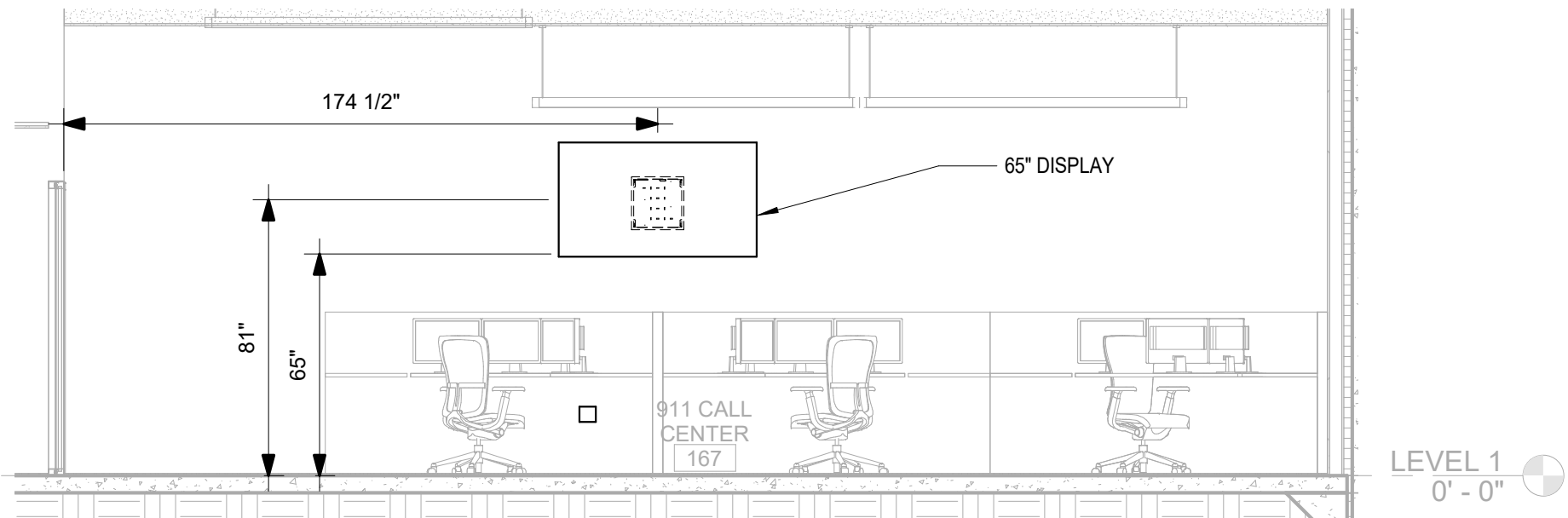
2 AV ELEVATION DETAILS - 911 CALL CENTER 167 - NORTH WALL 3 AV ELEVATION DETAILS - 911 CALL CENTER 167 - SOUTH WALL 1/4" = 1'-0" AV-302 AV-302
