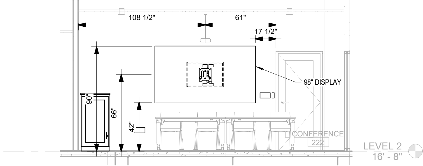
2 AV-303 AV ELEVATION DETAILS - CONFERENCE 222 1/4" = 1'-0"
