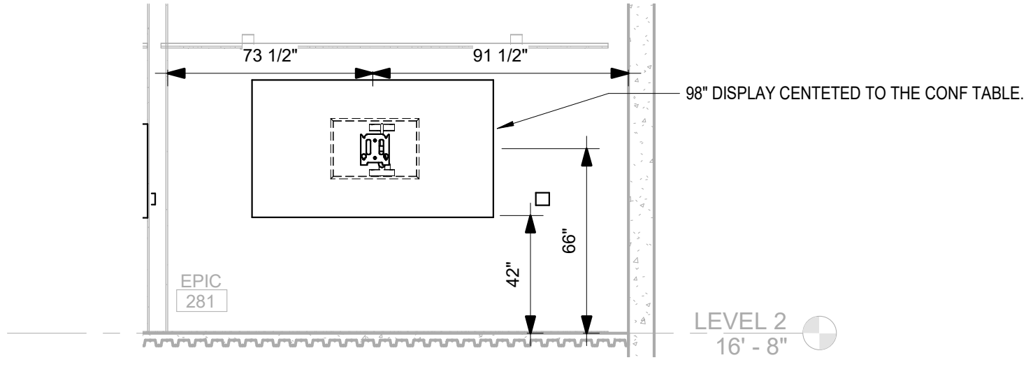
2 AV ELEVATION DETAILS - EPIC 281 1/4" = 1'-0" AV-305
