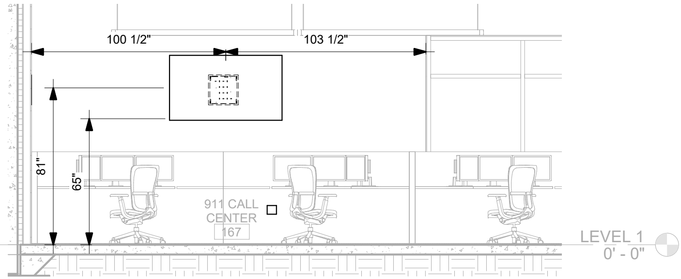
2 AV ELEVATION DETAILS - 911 CALL CENTER 167 - NORTH WALL 3 AV ELEVATION DETAILS - 911 CALL CENTER 167 - SOUTH WALL 1/4" = 1'-0" AV-302 AV-302
