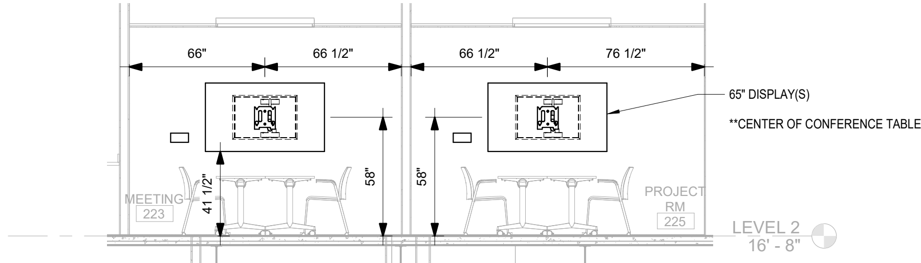
3 AV-303 AV ELEVATION DETAILS - MEETING / PROJECT RMS 1/4" = 1'-0"
