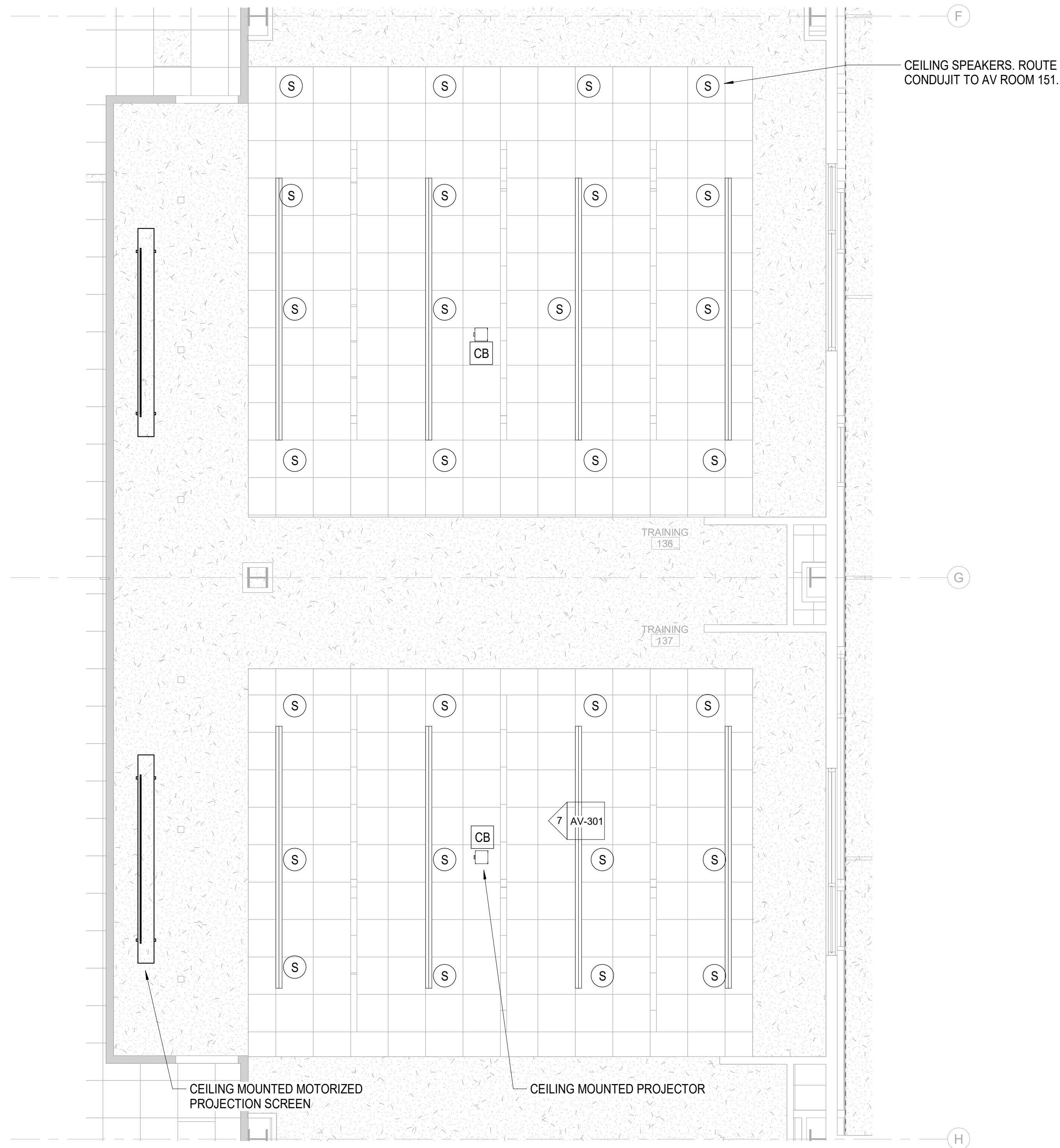
6 AV TRAINING ROOM(S) 137/137 - ENLARGED RCP PLAN AV-201 1/4" = 1'-0"
