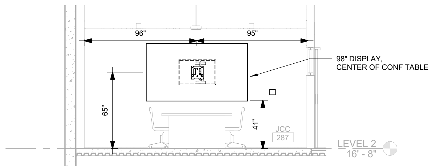
7 AV-305 AV ELEVATION DETAILS - JCC 287 1/4" = 1'-0"
