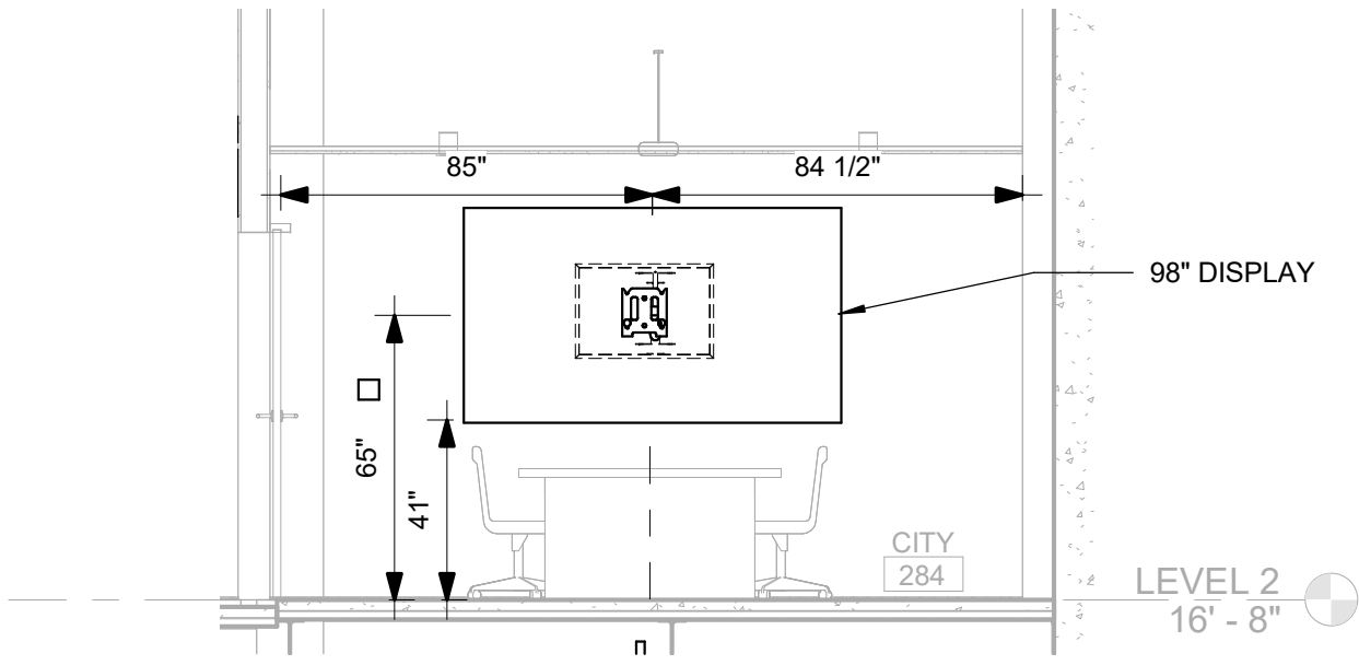
5 AV-305 AV ELEVATION DETAILS - CITY 284 1/4" = 1'-0"
