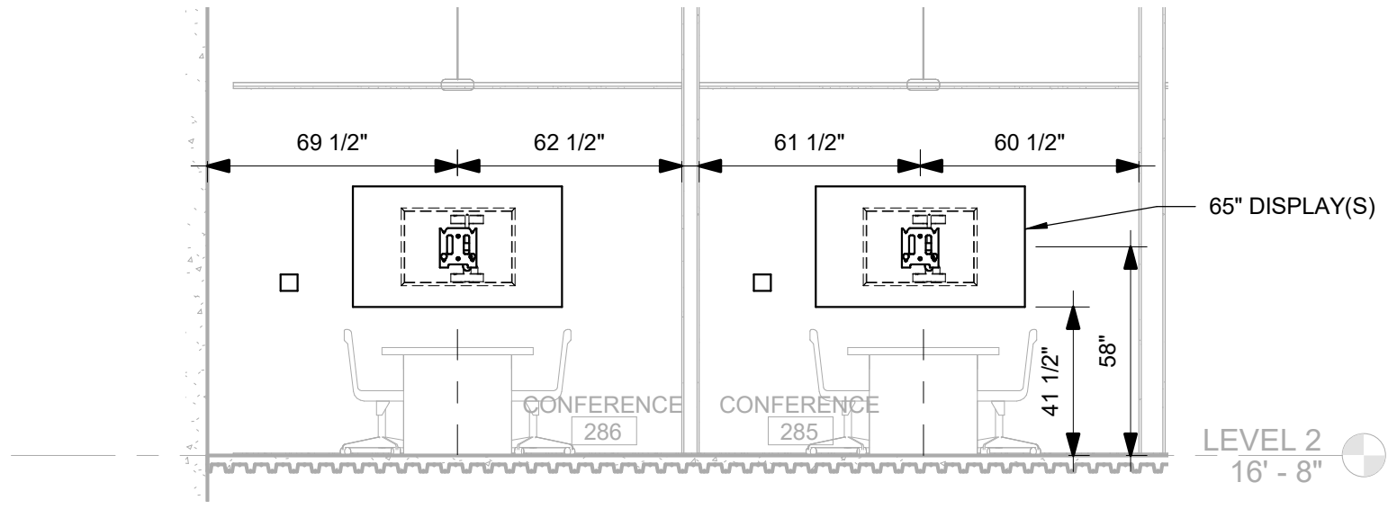
6 AV ELEVATION DETAILS - CONFERENCE ROOM 285 / 286 = 1'-0" AV-305
