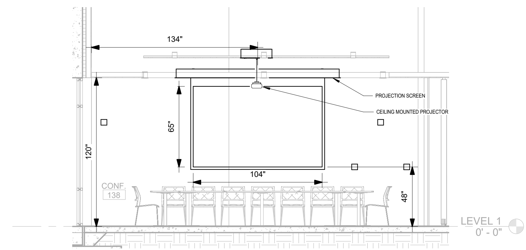
7 AV-301 AV ELEVATION DETAILS - PROJECTION SCREEN - PROJECTOR 1/4" = 1'-0" 8 AV-301 AV ELEVATION DETAILS - CONF 138 1/4" = 1'-0"
