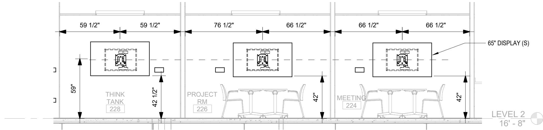
4 AV ELEVATION DETAILS - MEETING ROOM(S) AV-303
