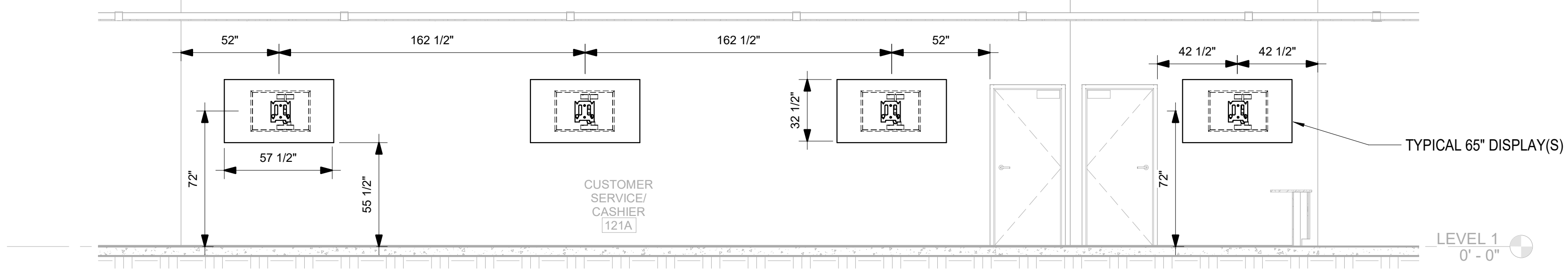
1 AV-301 AV ELEVATION DETAILS - VOTING MULTIPURPOSE 1544 = 1'-0" 2 AV-301 AV ELEVATION DETAILS - RECEPTION 154A 1/4" = 1'-0" 3 AV-301 AV ELEVATION DETAILS - CUSTOMER SERVICE / CASHIER 121 1/4" = 1'-0"
